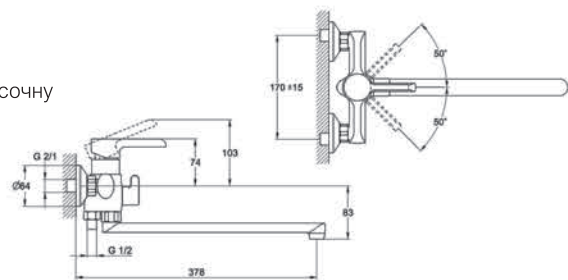
ЗМІШУВАЧ ДЛЯ ВАННИ З ПОВОРОТНИМ ВИЛИВОМ АРТИКУЛ: EZO7-A036YB
