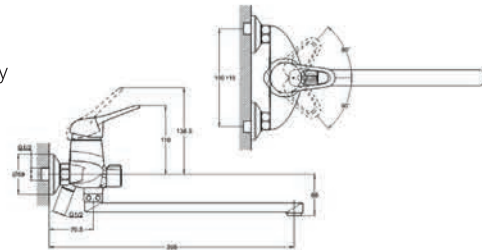
ЗМІШУВАЧ ДЛЯ ВАННИ З ПОВОРОТНИМ ВИЛИВОМ 320MM АРТИКУЛ: NHK7-A048
