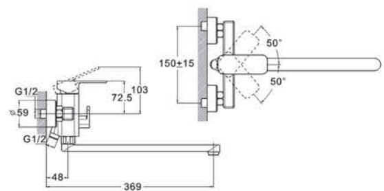
ЗМІШУВАЧ ДЛЯ ВАННИ З ПОВОРОТНИМ ВИЛИВОМ АРТИКУЛ: LEB7-B123
