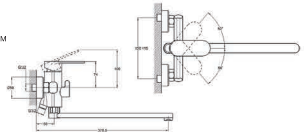
ЗМІШУВАЧ ДЛЯ ВАННИ З ЛИТИМ ПОВОРОТНИМ ВИЛИВОМ АРТИКУЛ: LOB7-A128
